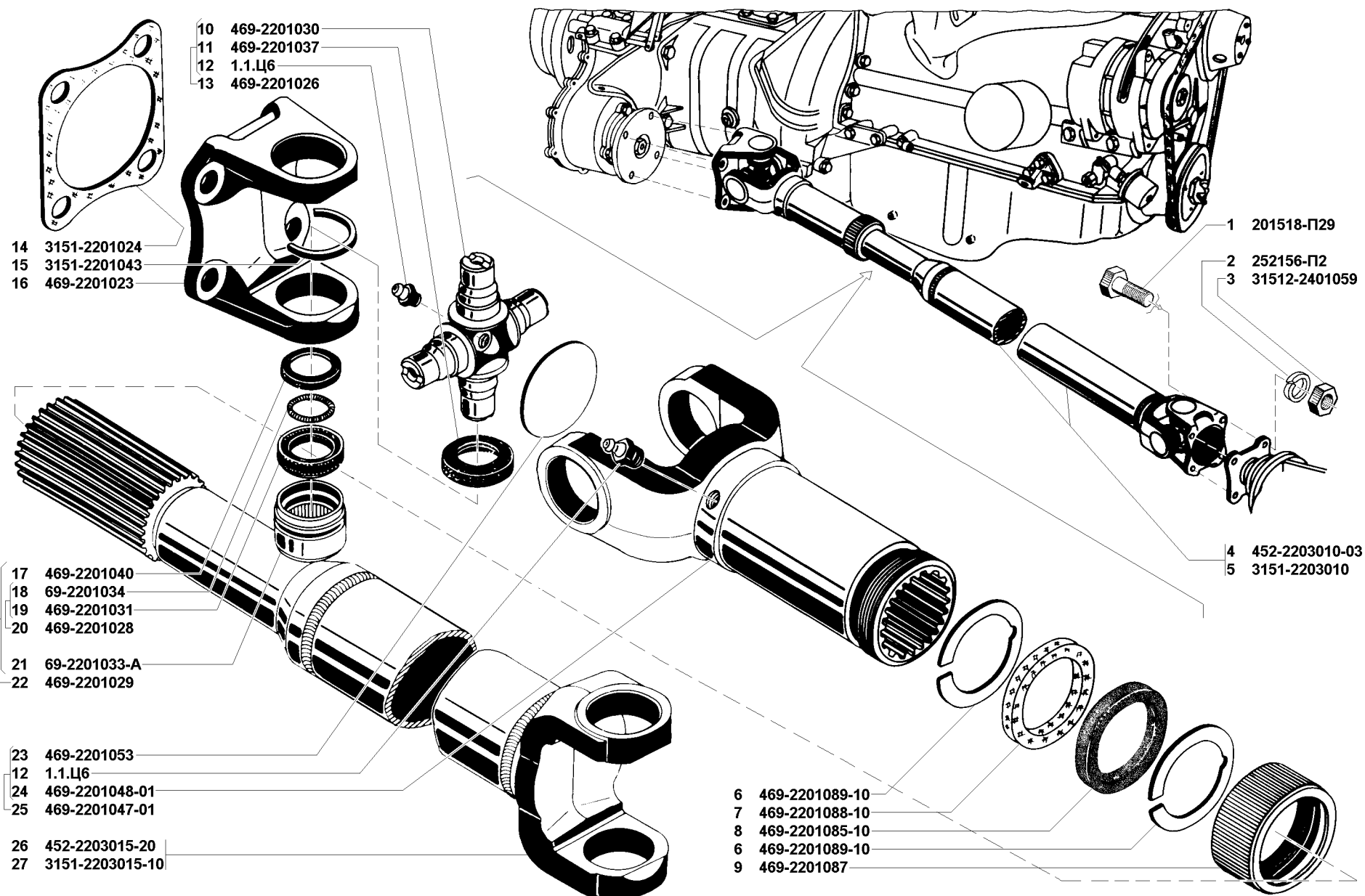
Рис. 57. Вал карданный переднего моста (2203) Fig. 57. Front axle propeller shaft (2203)
